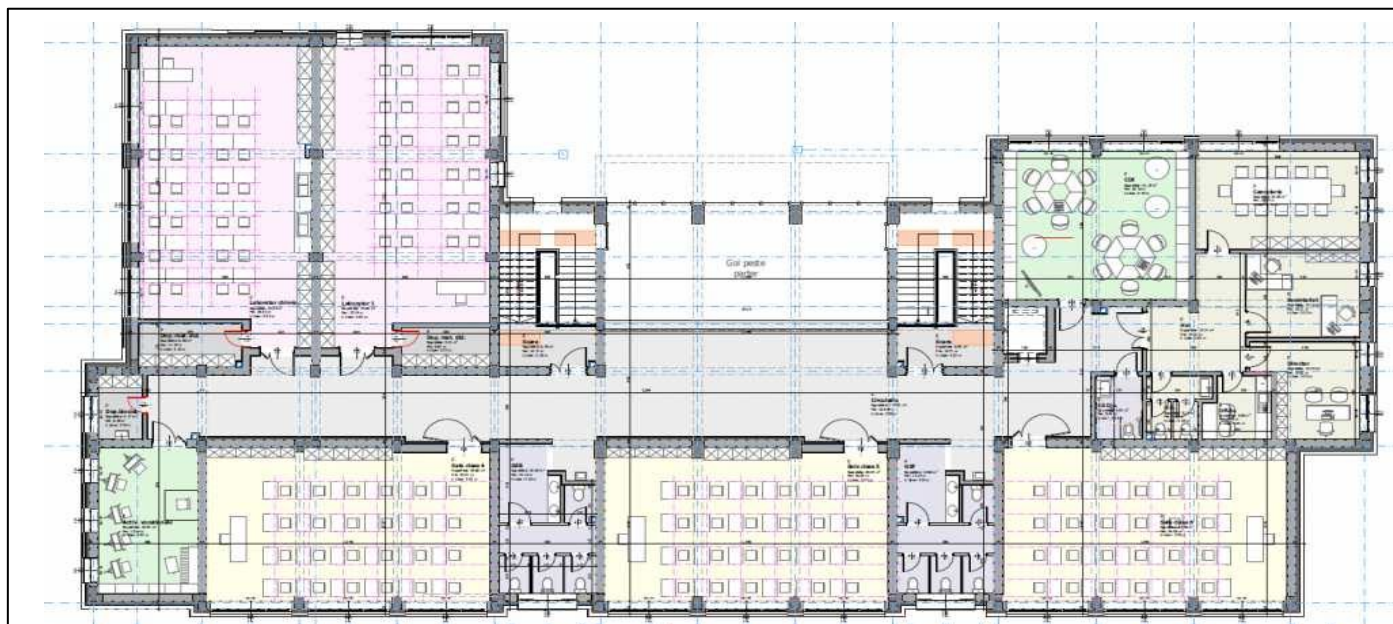
Fig. 6. Planul propus pentru noua construcție (etaj)
