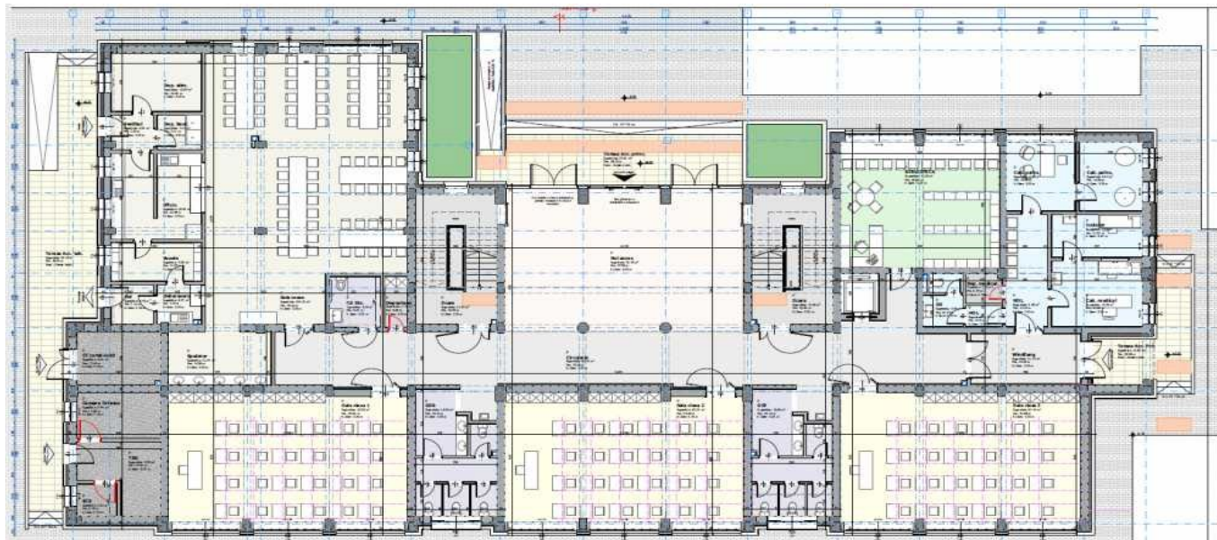
Fig. 5. Planul propus pentru noua construcție (parter)
